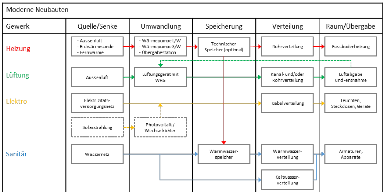
Abbildung 20: Schematische Darstellung der Gebäudetechniksysteme eines modernen Neubaus mit Unterteilung der Teilprozesse nach SIA 411
