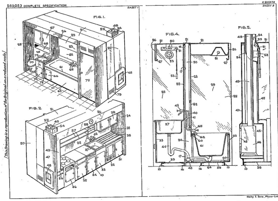
Abbildung 22: Beispiel «Raummodul», Patentrecherche GB569053A
