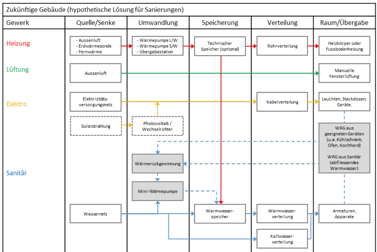
Abbildung 21: Schematische Darstellung der Gebäudetechniksysteme von zukünftigen Gebäuden (hypothetische Lösung für Sanierungen) mit Unterteilung der Teilprozesse nach SIA 411
