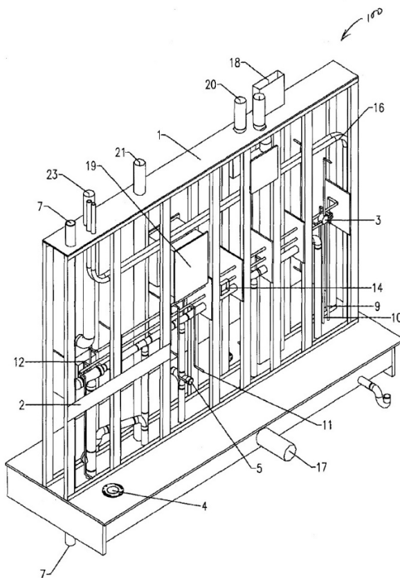
Abbildung 23: Beispiel «Steigzone», Patentrecherche US2010229472A1 (16.09.2010)
