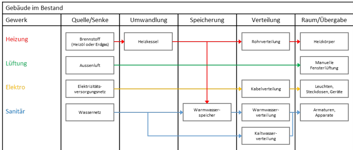
Abbildung 19: Schematische Darstellung der Gebäudetechniksysteme eines typischen Gebäudes im Bestand mit Unterteilung der Teilprozesse nach SIA 411
